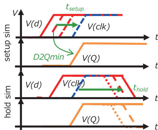
図. フリップフロップのキャラクタライズ例。対象となるセルの入力波形の生成と、出力波形の読み取り、ライブラリ生成を自動で行う。
