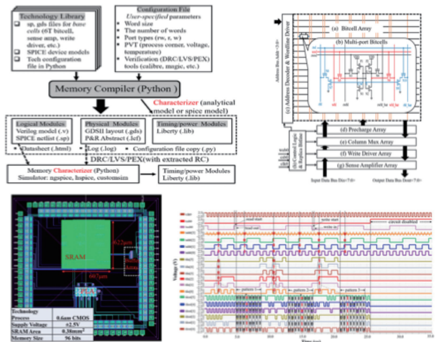
図. OpenRAM を活用した試作事例
