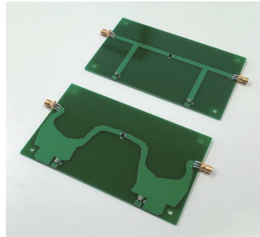
図. 導体レイアウトの最適設計 (手前:最適なレイアウト 奥:一般的レイアウト)
