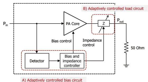
図. Power Amplifier のアーキテクチャ
