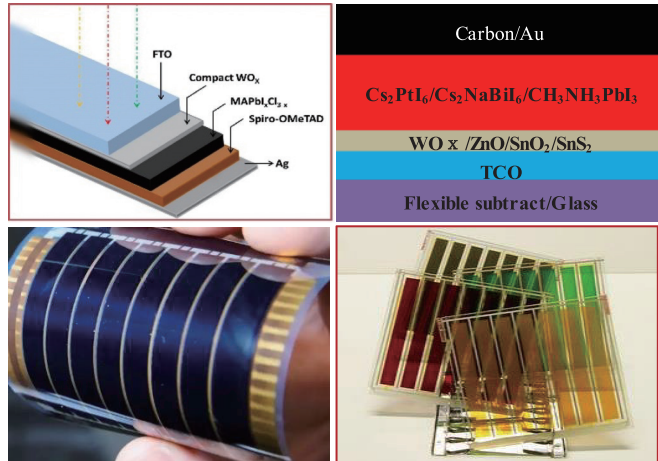
図. 開発した光電デバイス
