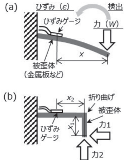
図. センサー変形前後の構造
