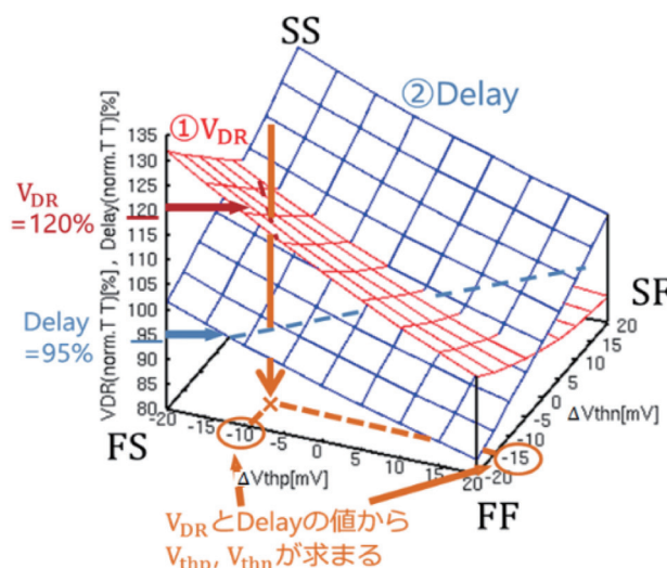
図. フリップフロップの記憶保持特性と RO 周波数・IDDQ などから、ばらつき量( \Delta V_{th,N} , \Delta V_{th,P} )を推定する
