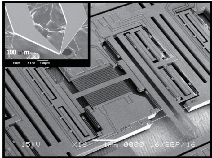
図. MEMSピンセット、左上は微小物質を把持するプローブ部分の拡大
