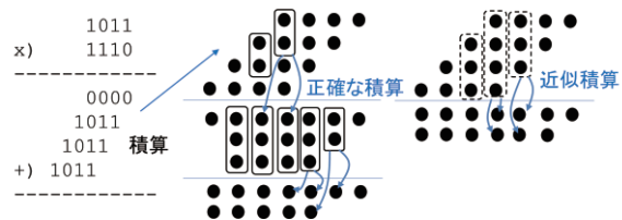
図. データ表現と演算器の最適化
