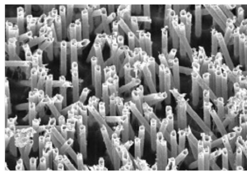
Fig. 2 SEM image of Au nanostraw membrane.
