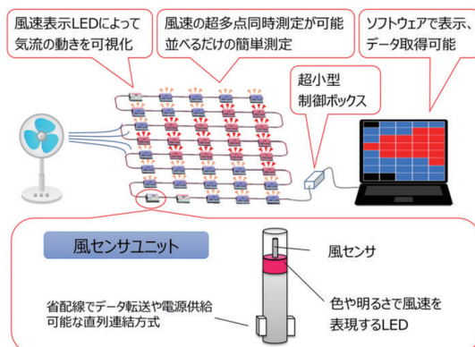
新たな取り組み(気流計測ユニット)
