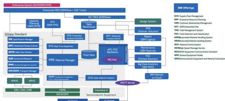
SiViewシステム構成イメージ
