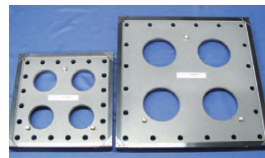
ホールプレート（3次元測定機校正用）
