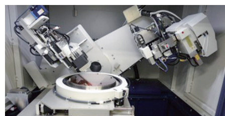
X線トポグラフ装置 (XRTmicron)
