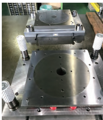
モータコア金型
